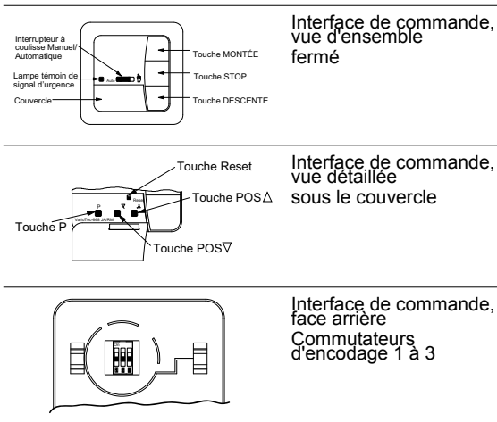
Fig. 1 Vues de l'appareil
