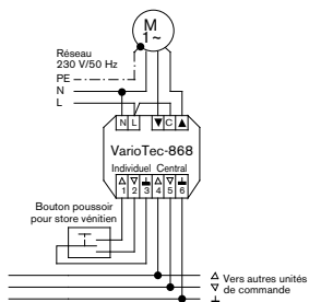
Fig. 3 Connexion comme appareil de commande d'entraînement
