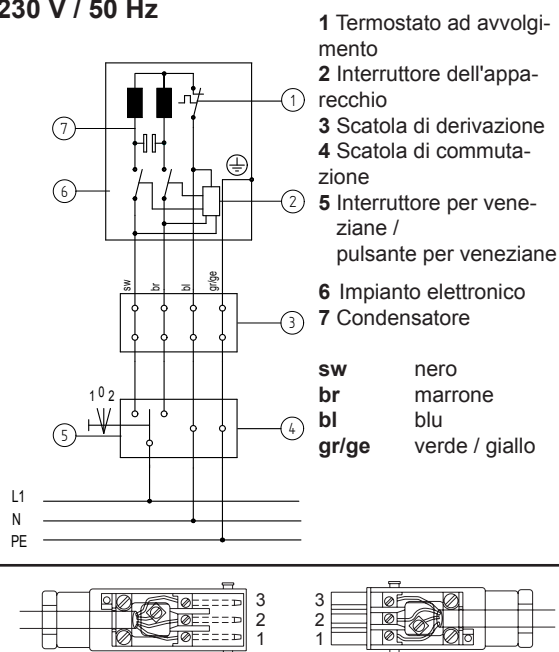
Fig. 5 Schema elettrico di SunTop/Z M RH con 230 V / 50 Hz ed assegnazione dei cavi con l'impiego con il collegamento ad innesto Hirschmann STAS-3
