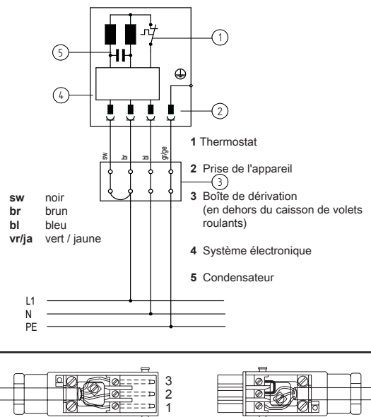
Fig. 5: Plan de câblage SunTop/Z M-868 RH 230 V / 50 Hz et pose du câble avec raccord enfichable Hirschmann STAS-3 (avec pont)
