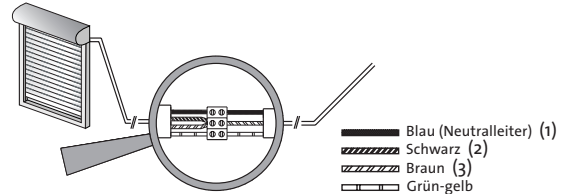
Fig. 7: Raccordement radio (mode émetteur)
