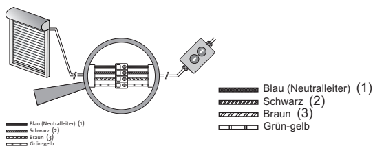
Fig. 6 Allacciamento per i cavi di montaggio
