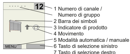
Fig. 1 Display in modalità di funzionamento (Esempio 1): Canale 12, veneziana programmata, modalità automatica attiva, movimento salita
